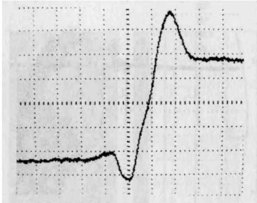
Рис. Г8 - Реальные эпюры напряжения от телекамеры в точке 4. (см. Рис. Г3) Переходная характеристика с черного фона на белый.
