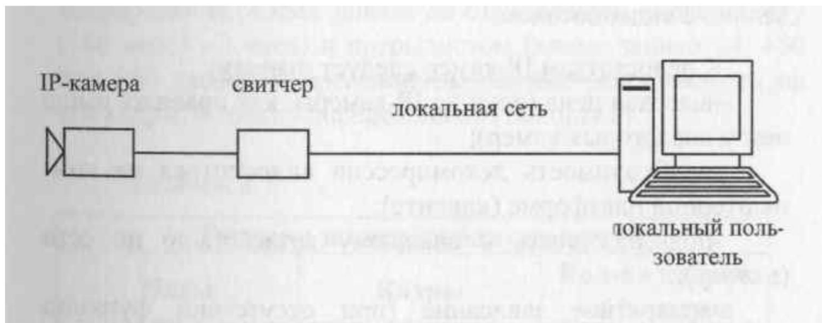
Рис. 11 - Схема работы IP-камер в локальной сети
