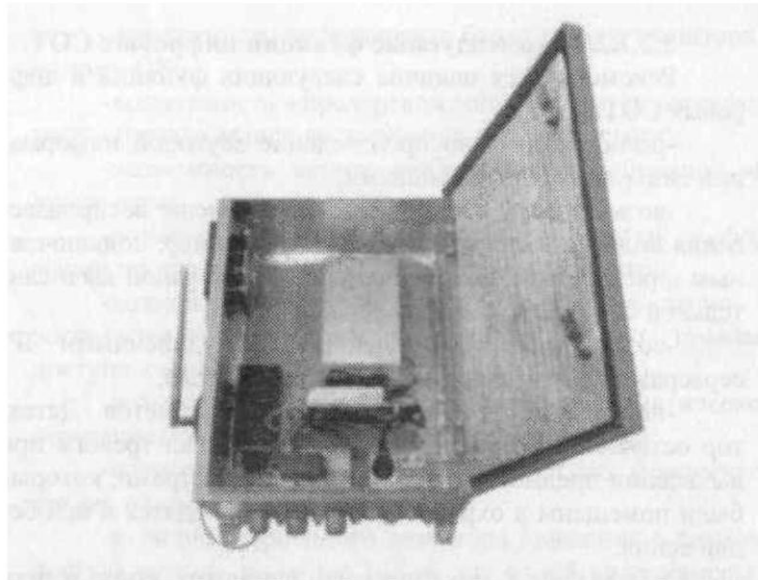
Рис. 8 - Удаленный IP-видеосервер в термокожухе с возможностью взаимодействия через WiFi канал.
