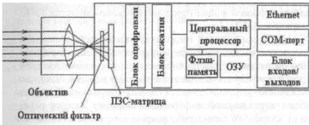
Рис. 10- Устройство IP-камеры
