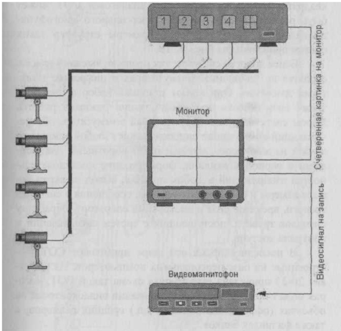
Рис. 17 Структурная схема системы видеонаблюдения с квадратором
