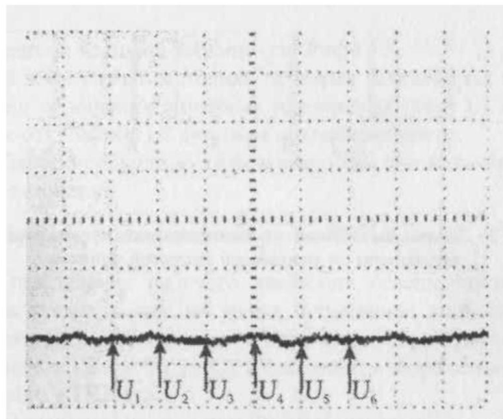
Рис. Г5 - Реальные эпюры напряжения от телекамеры в точке 2 (см. Рис. Г3)
