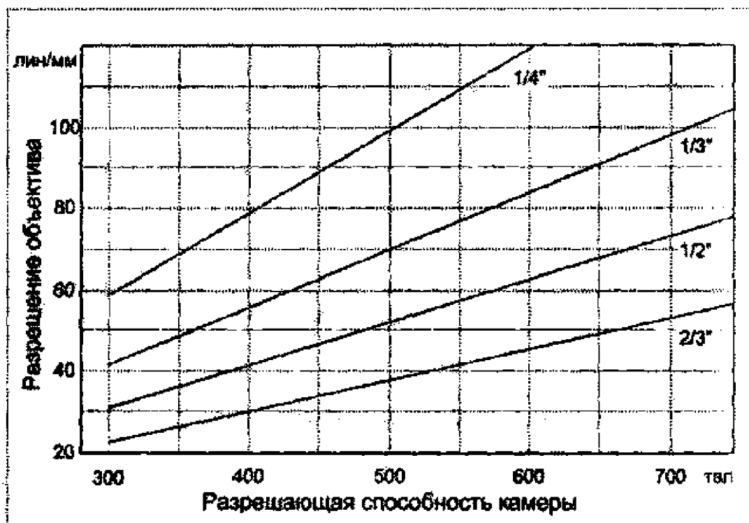
Рис. Ж1 - Необходимое разрешение объектива в зависимости от ширины диагонали матрицы камеры
