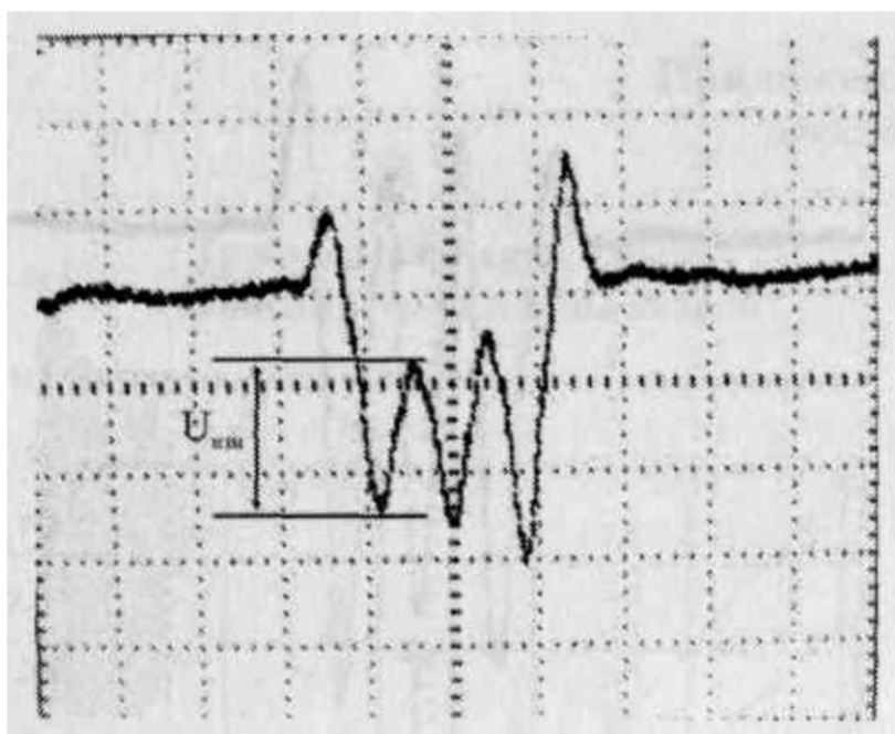
Рис. Г11 - Реальные эпюры напряжения от телекамеры в точке 8 (см. Рис. ГЗ)
