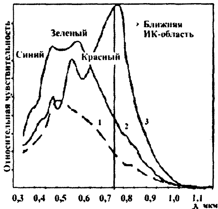
Рис. А2 - Спектральные характеристики чувствительности ПЗС:
