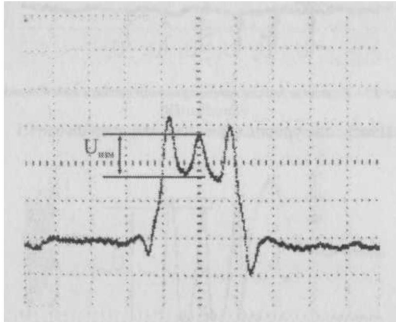
Рис. Г4 - Реальные эпюры напряжения от телекамеры в точке 1 (см. Рис. Г3) Измерение разрешения в СОТ с помощью штриховой миры (визуальная оценка глубины модуляции).
