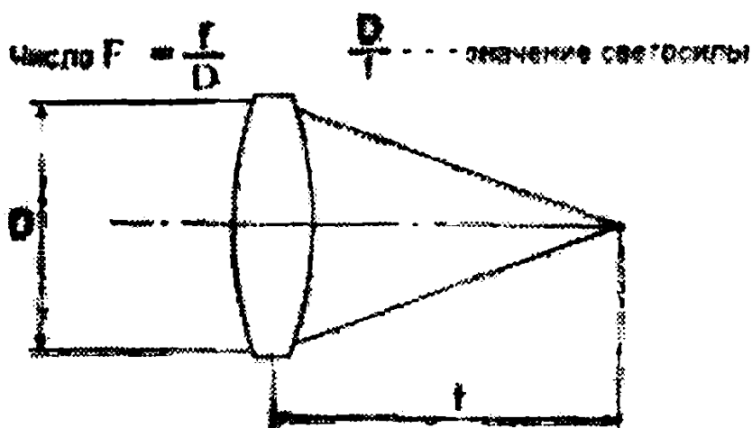
Рис. А3 - Светосила объектива
