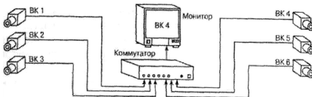
Рис. 16 - Структурная схема системы видеонаблюдения с коммутатором
