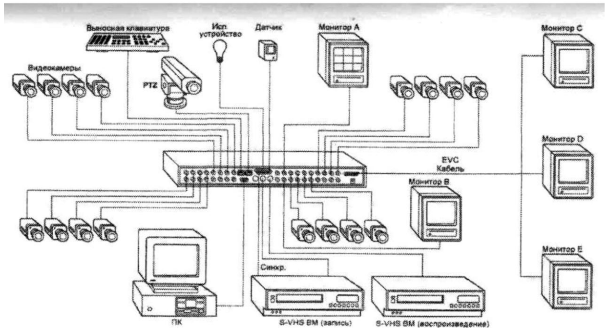
Рис.18 - Структура СОР на базе универсального мультиплексора
